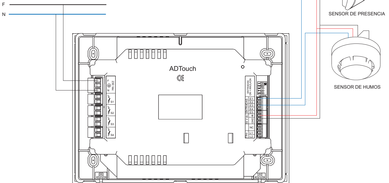
Esquema de instalación con sensores externos opcionales
