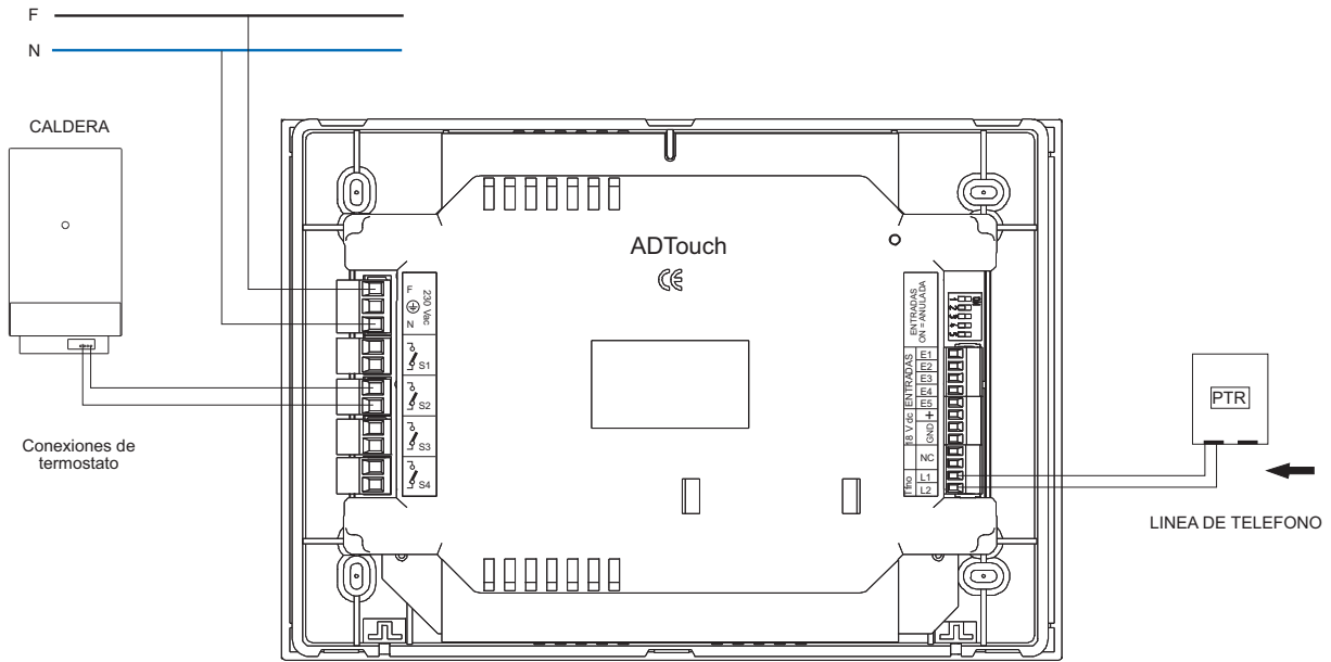
Esquema de instalación básica
