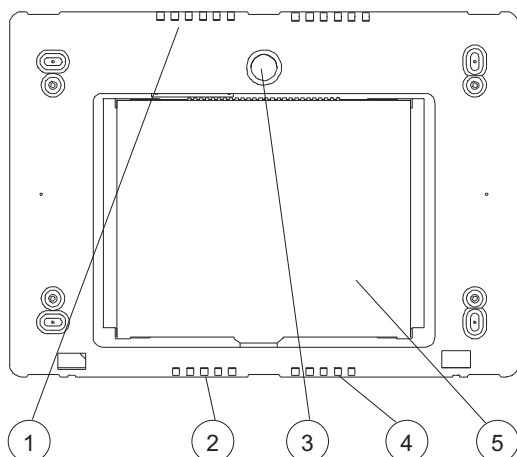
Vista frontal sin el marco embellecedor. Identificación de los elementos característicos de ADTouch y su ubicación.
