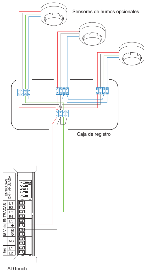
Esquema de instalación con sensores externos opcionales
