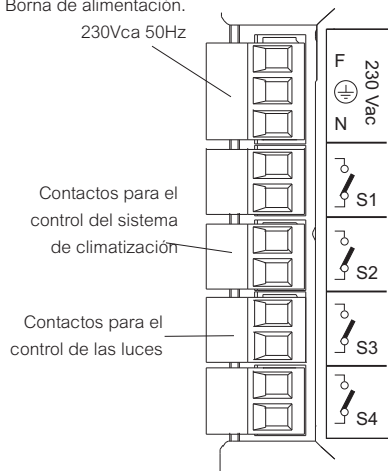
Detalle de las bornas de las salidas a relés. Contactos libres de potencial
