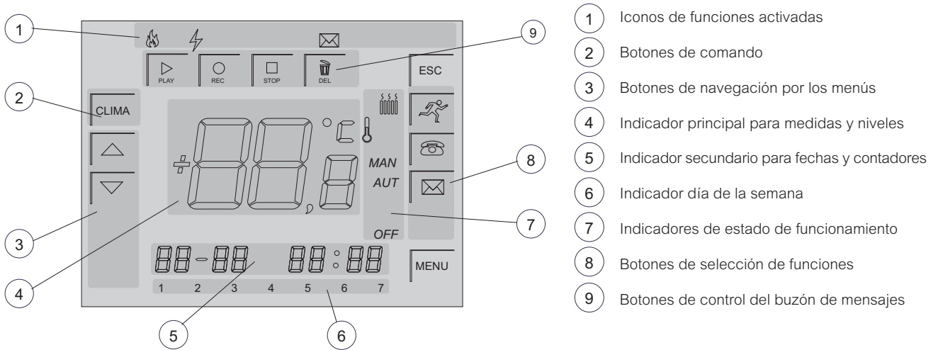
Ubicación de elementos de control y visualizadores de la pantalla LCD Touch
